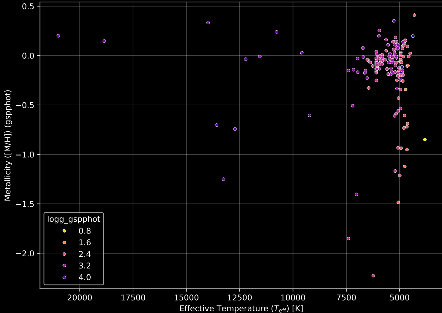
APOGEE DR17 Field: [143+04] Stellar Population Parameters (n= 178)
